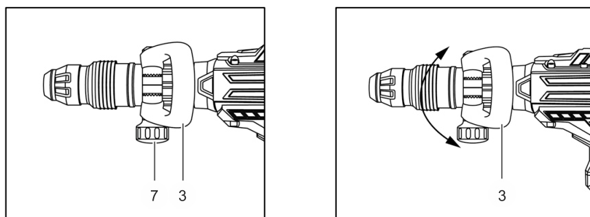
Рис. 2. Установка дополнительной рукоятки
