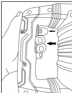
Рис. 5. Нажатие кнопки фиксации включателя
