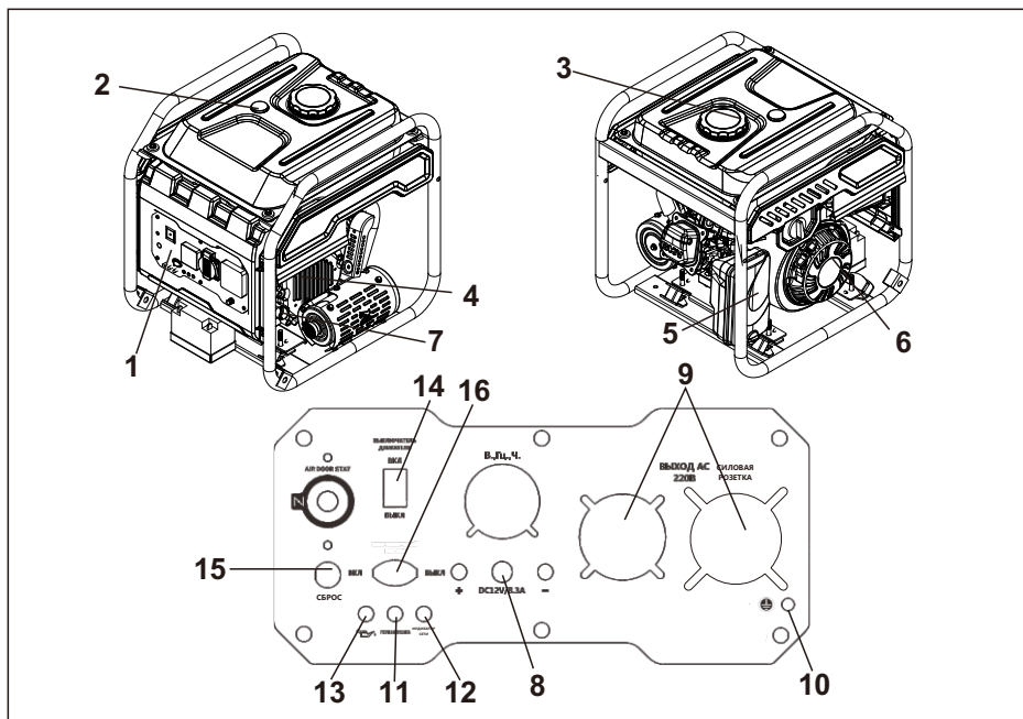
Рис.10 Общий вид модели BR750iOL
