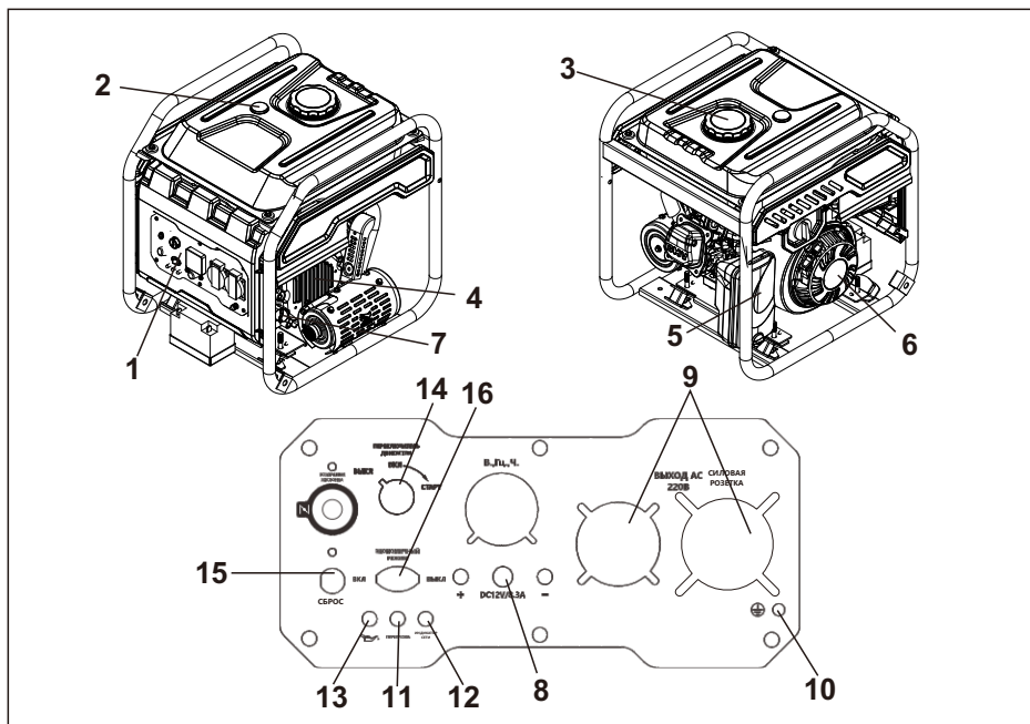
Рис.11 Общий вид модели BR7500iOEL
