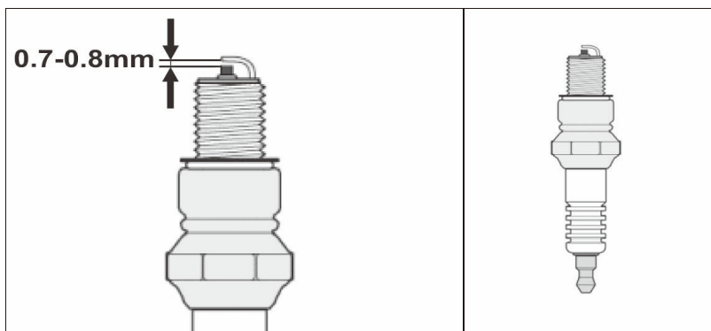
Рис. 15. Свеча зажигания
