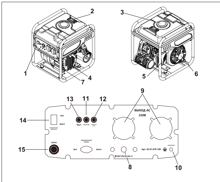
Рис.9 Общий вид модели BR7500iO
