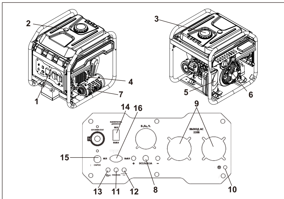
Рис.7 Общий вид модели BR5000iOL
