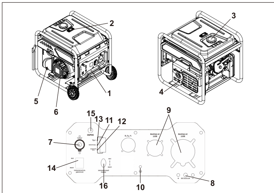
Рис.12 Общий вид модели BR8500iOM
