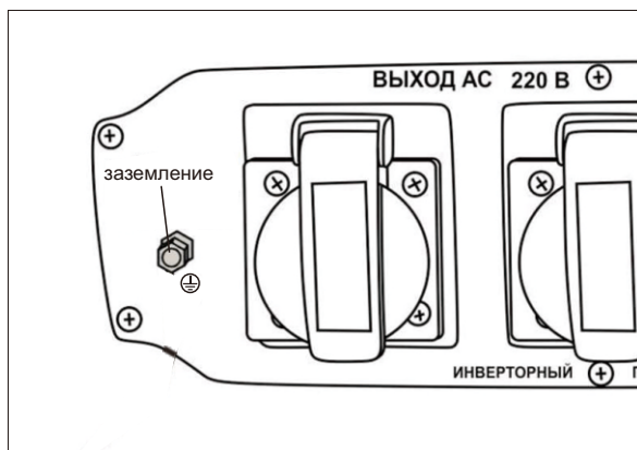
Рис. 6. Заземление
