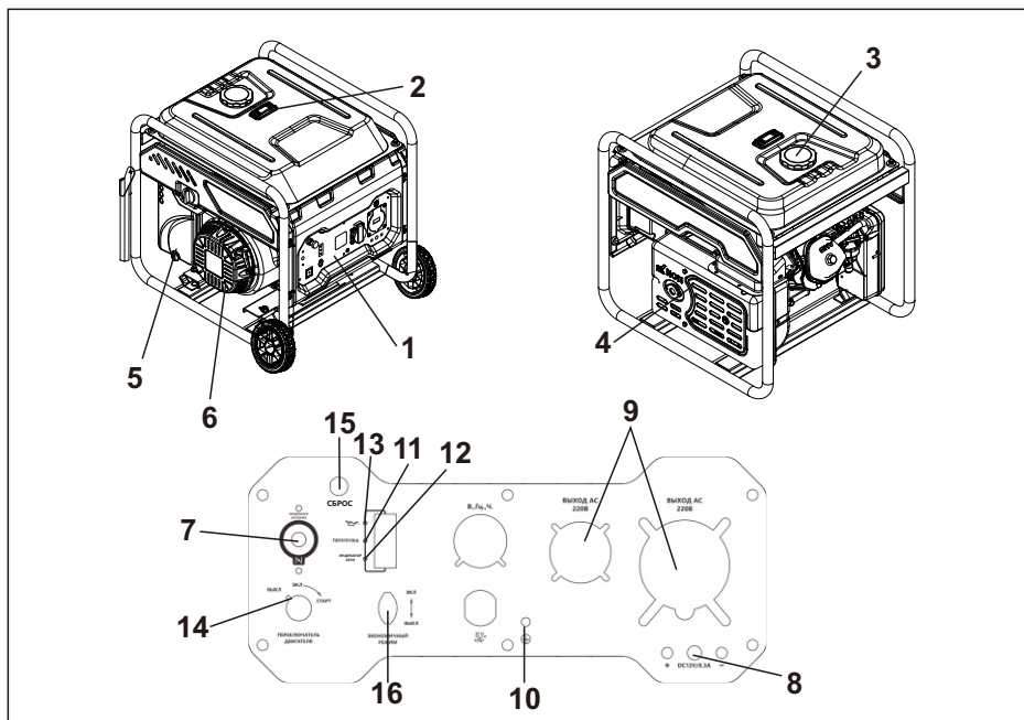
Рис.13 Общий вид модели BR8500iOEM
