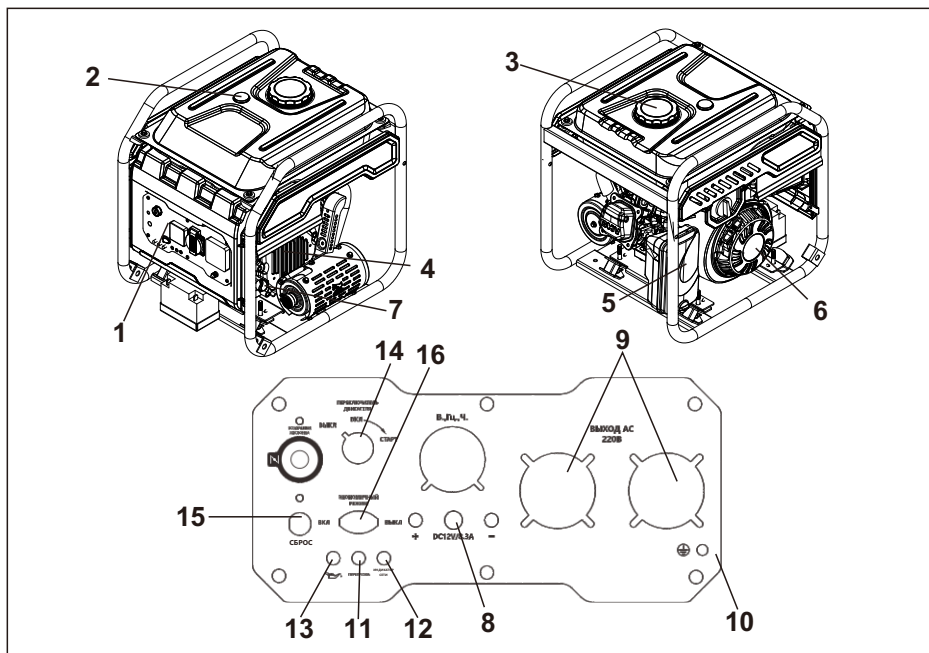
Рис.8 Общий вид модели BR5000iOEL
