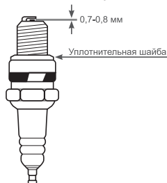
Рис. 14 Обслуживание свечи зажигания
