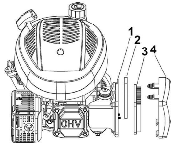
Рис. 12 Обслуживание воздушного фильтра
