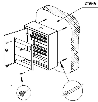
Рис.1. Схема монтажа
