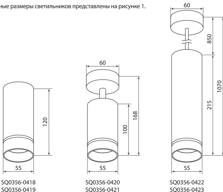
Рисунок 1. Габаритные размеры светильников, мм
