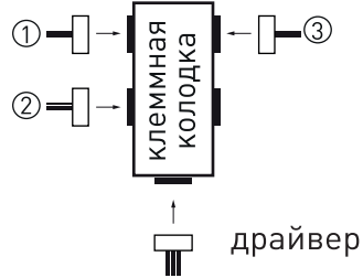
(Рис. 2) Соединение проводов согласно маркировки
