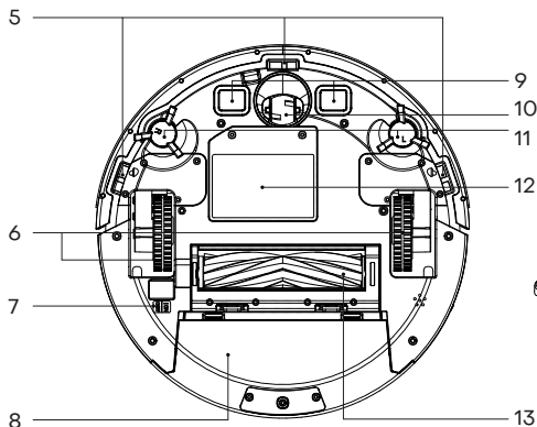
Вид снизу
