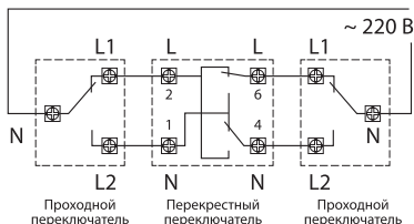
Рисунок 4. Схема подключения перекрестного выключателя.
