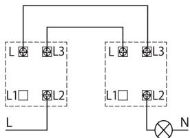
Рисунок 3. Схема подключения проходного выключателя.
