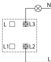
Рисунок 1. Схема подключения одноклавишного выключателя.
