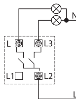
Рисунок 2. Схема подключения двухклавишного выключателя.
