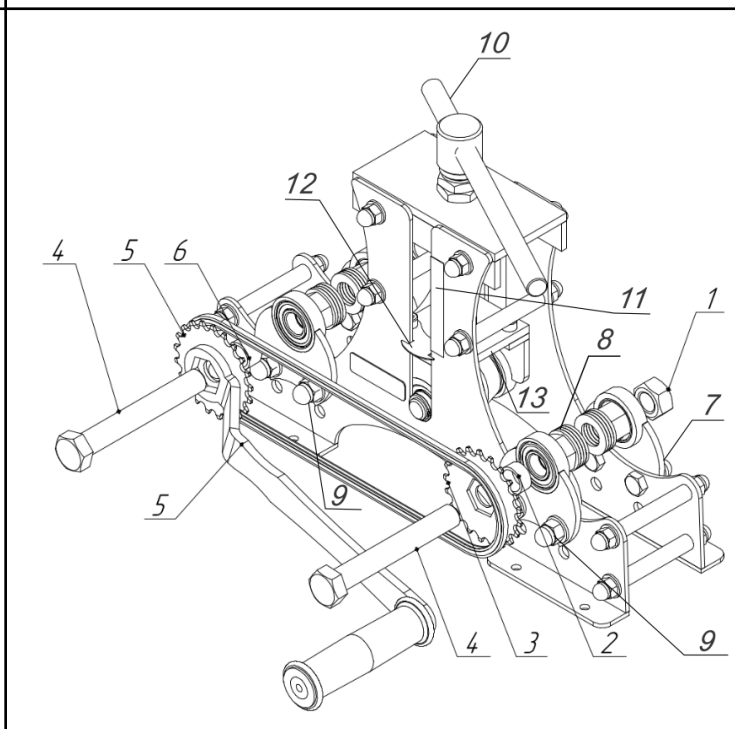
Рис. 4. Профилегипб "удачный Стандарт"
