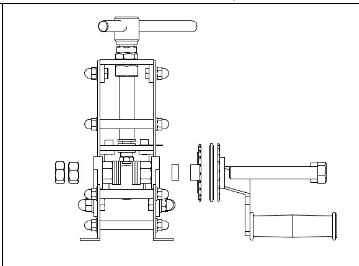
Рис. 2 Профилегипб "удачный Стандарт". Вид сбоку
