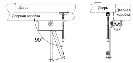
Стандартная установка доводчика на дверную коробку
