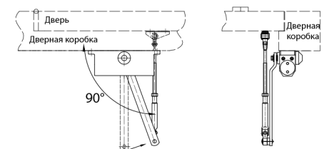
Стандартная установка доводчика на дверную коробку
