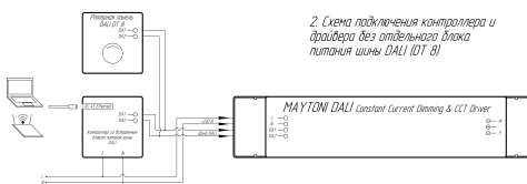
3. Схема подключения контроллера и драйвера с отдельным блоком питания шины DALI (DT 8)
