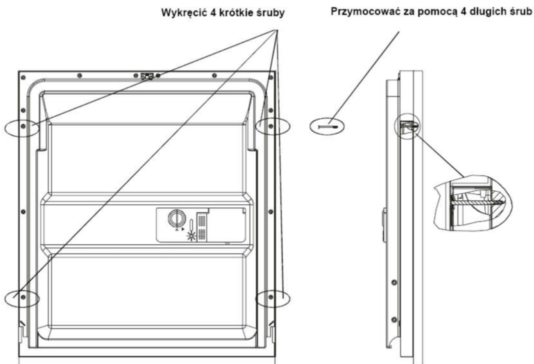
[Rysunek 4b] Montaż ozdobnego panelu meblowego
