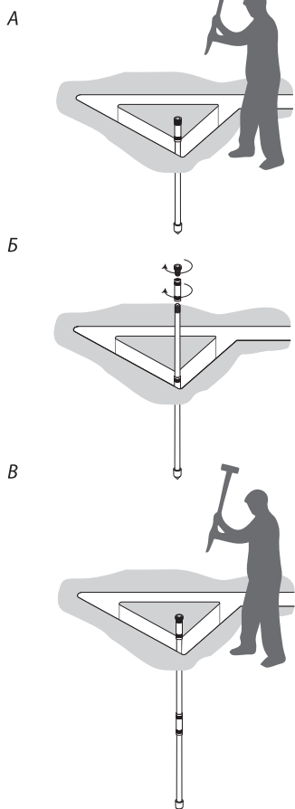
Рисунок 4. Этапы монтажа очага заземления
