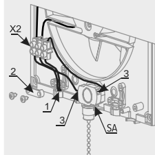
6 ші сурет OPTIMA (-02 опциясы)
