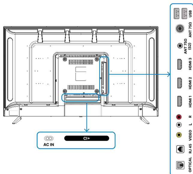
Рисунок 1 – Терминалы задней панели телевизора
