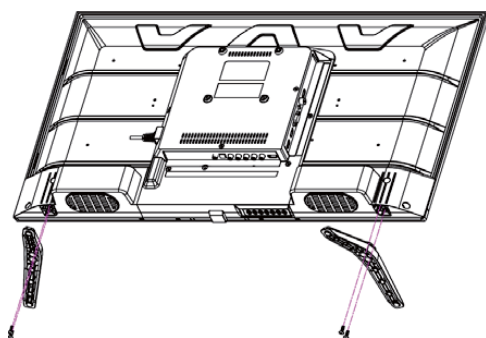
Комплект винтов для крепления подставок
