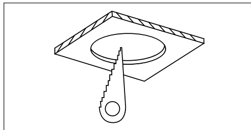
Рисунок 2. Подготовьте отверстие
