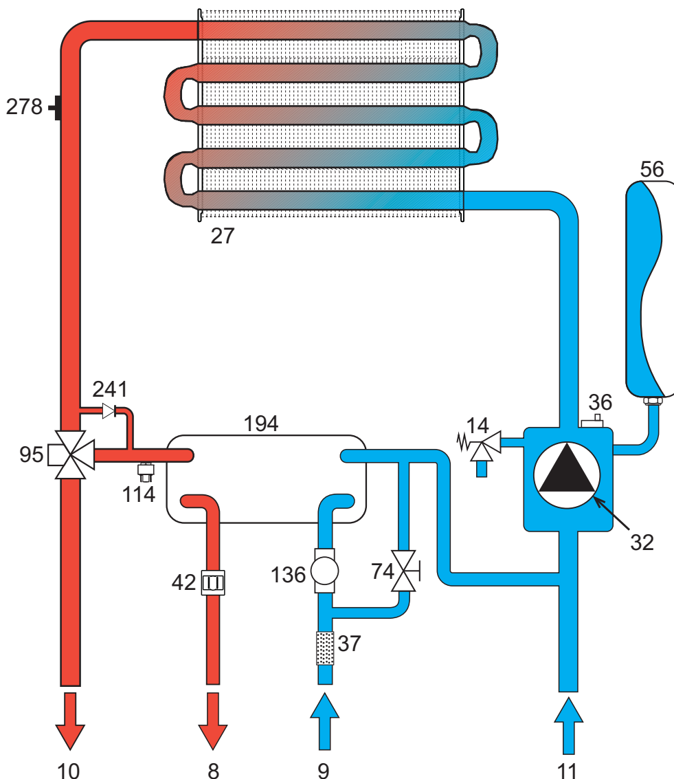
рис. 36- Контур отопления
