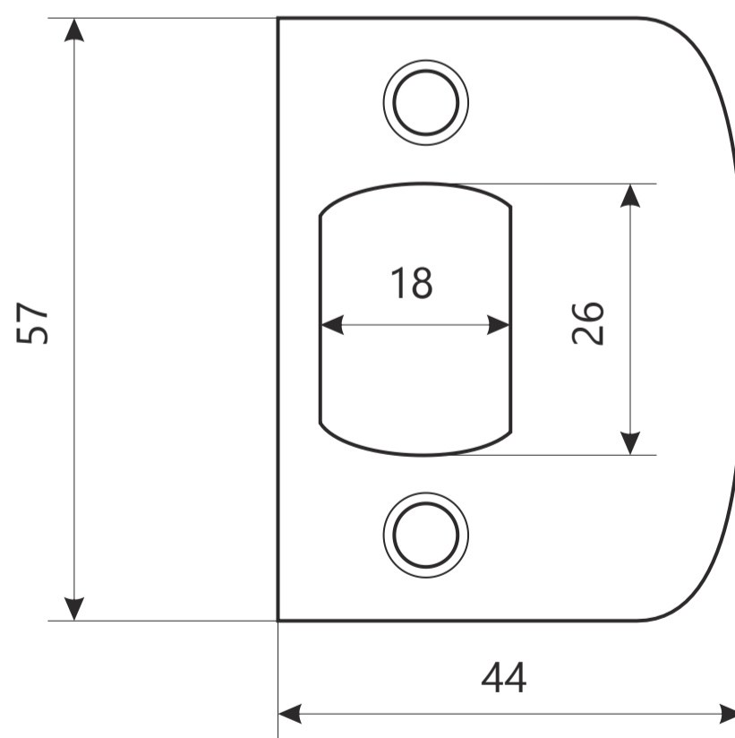
Ответная планка
