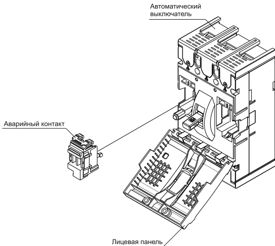
Рисунок 3 – Установка устройств в выключателе BA88 серии MASTER
