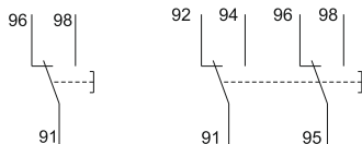
Рисунок 2 – Электрическая схема устройства
