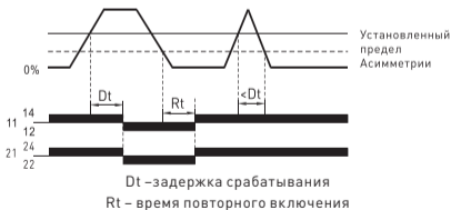
Рис. 3 – Принцип работы реле при асимметрии напряжения
