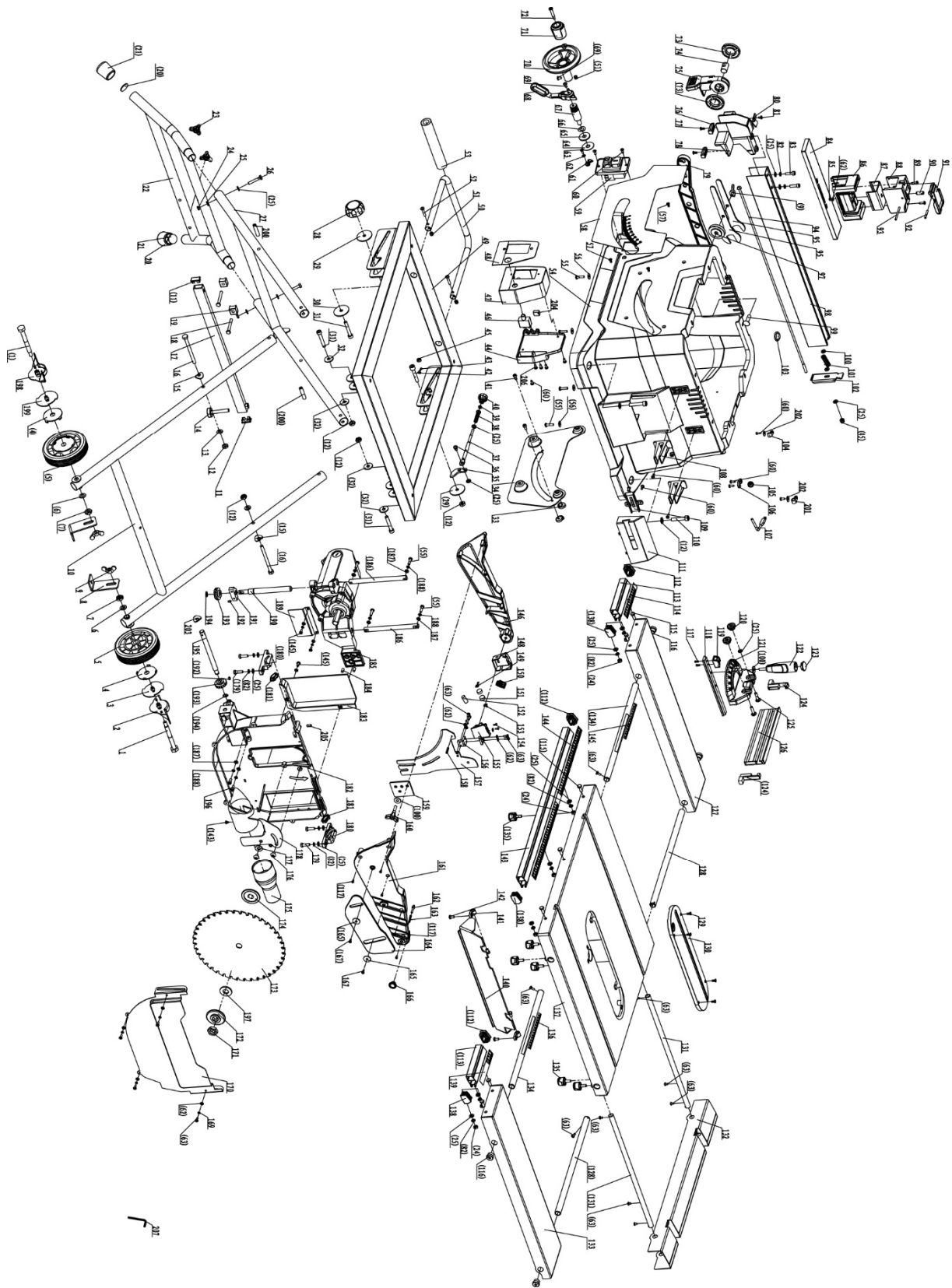
Рисунок 30. Взрыв-схема станка
