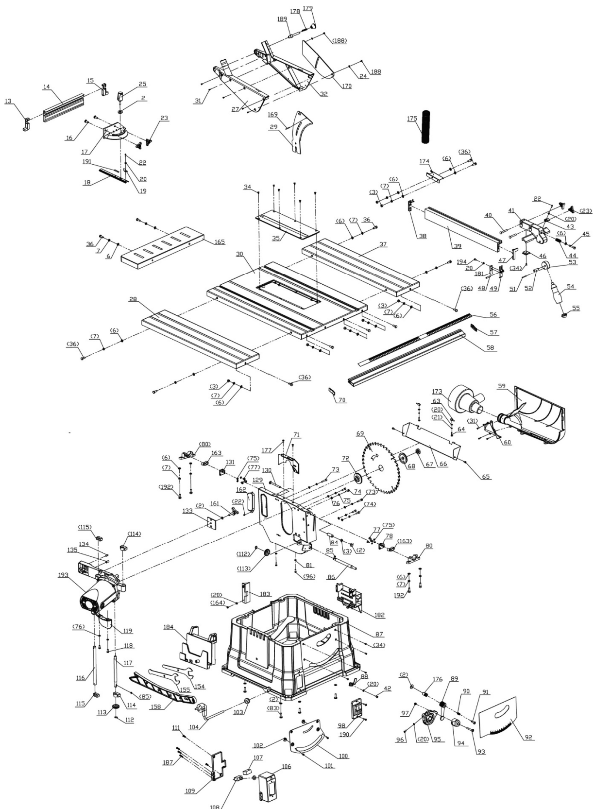
Рисунок 30. Взрыв-схема станка
