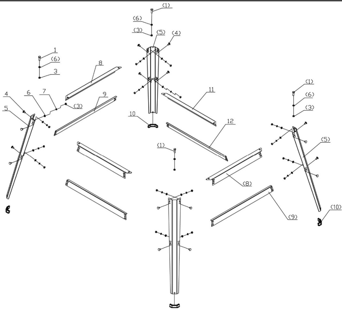
Рисунок 31. Взрыв-схема основания
