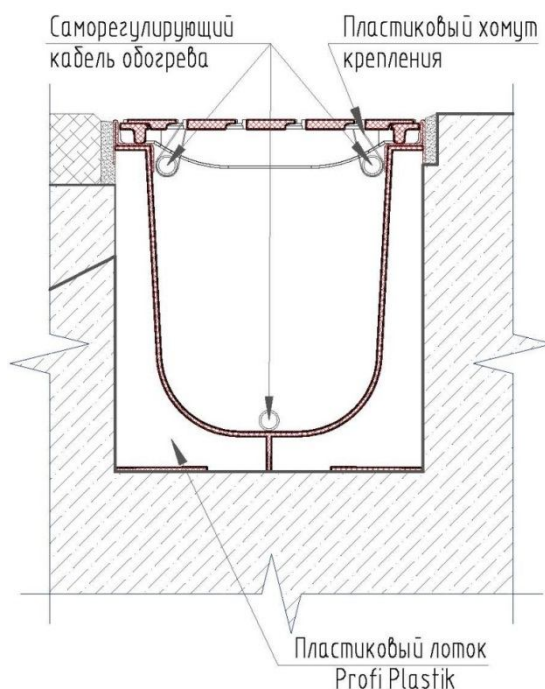
Рис. 4 – Схема монтажа устройства защиты от обледенения лотка.
