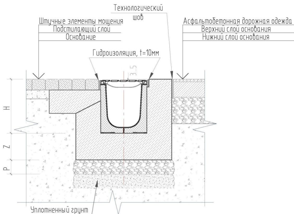
Рис. 6а – Монтаж пластиковых лотков с асфальтобетонным покрытием и штучными элементами мощения.
