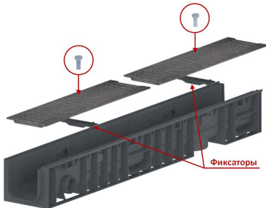
Рис. 2 – Лоток серии Norma Plastik (решетка крепится при помощи фиксаторов).
