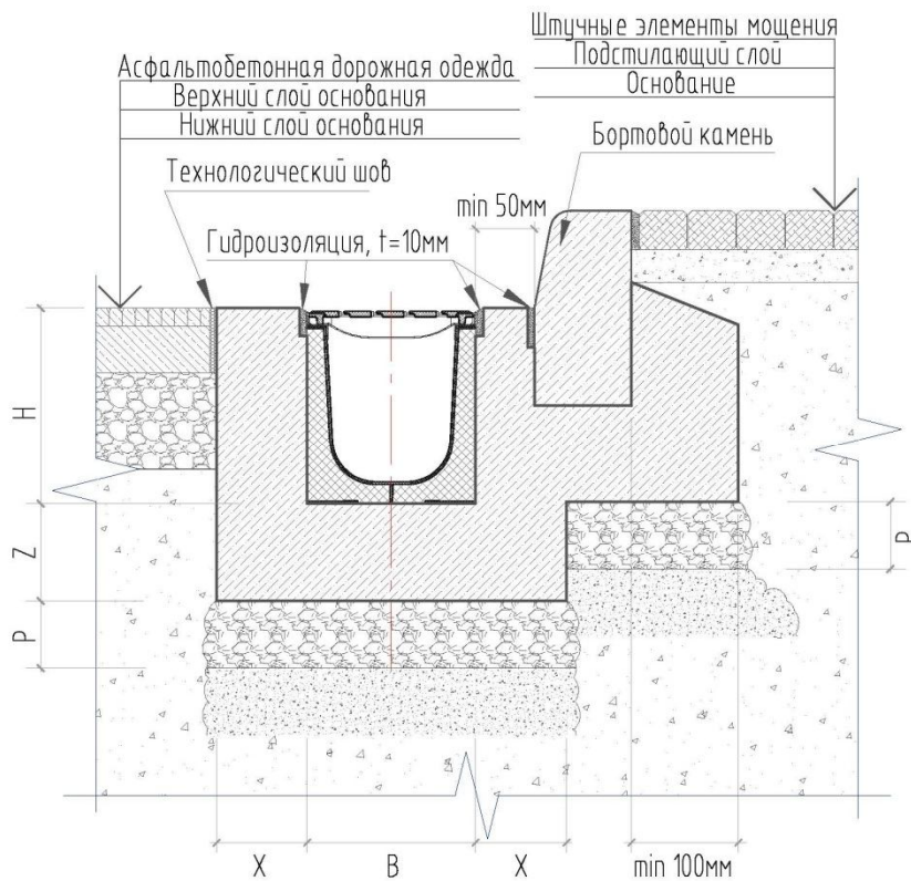
Рис. 7 – Монтаж пластиковых лотков с асфальтобетонным покрытием и бортовым камнем.
