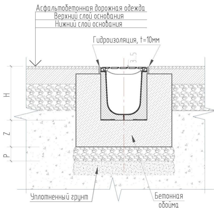
Рис. 6б – Монтаж пластиковых лотков с асфальтобетонным покрытием.
