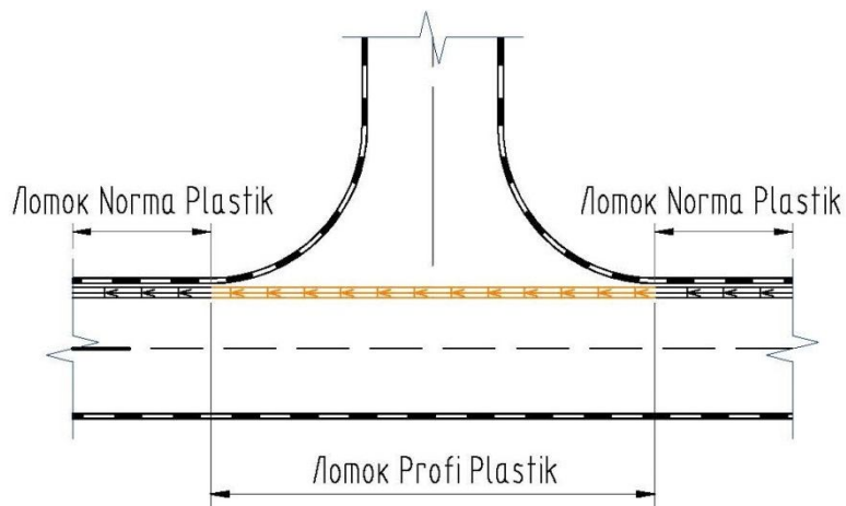
Рис. 1а – Участок дороги с переездом через линию водоотвода.
