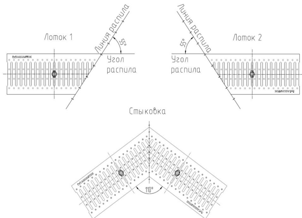
Рис. 10 – Пример стыковки распиленных лотков.
