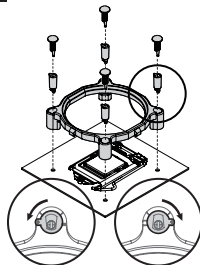
LGA 1700
