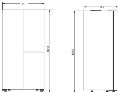
Модель CS5073FV
