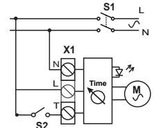
Схема электрическая 3
