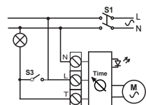
Схема электрическая 4
