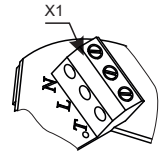
Схема монтажная
