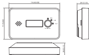
Figura 3-1 Dimensiones (mm[inch])
