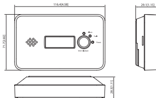
Abbildung 3-1 Abmessungen (mm)
