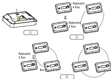
Figure 5-1 Interconnecter l'appareil
