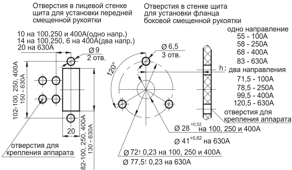
Рисунок В.2 – Расположение отверстий в стенках щита.
