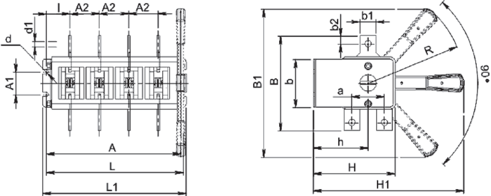
Рисунок 5.20 –Выключатель-разъединитель четырехполюсный на два направление с боковой рукояткой.
