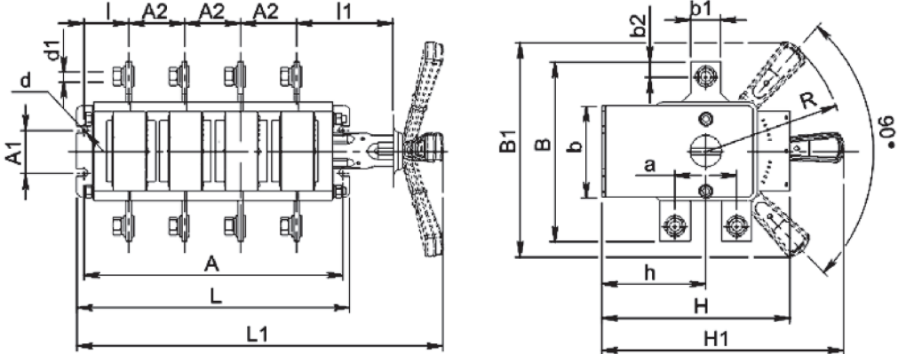
Рисунок 5.22 –Выключатель-разъединитель четырехполюсный на два направление с боковой смещенной рукояткой.
