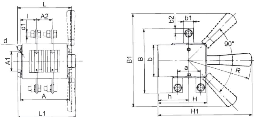
Рисунок Б.12 – Выключатель-разъединитель двухполюсный на два направления с боковой рукояткой.
