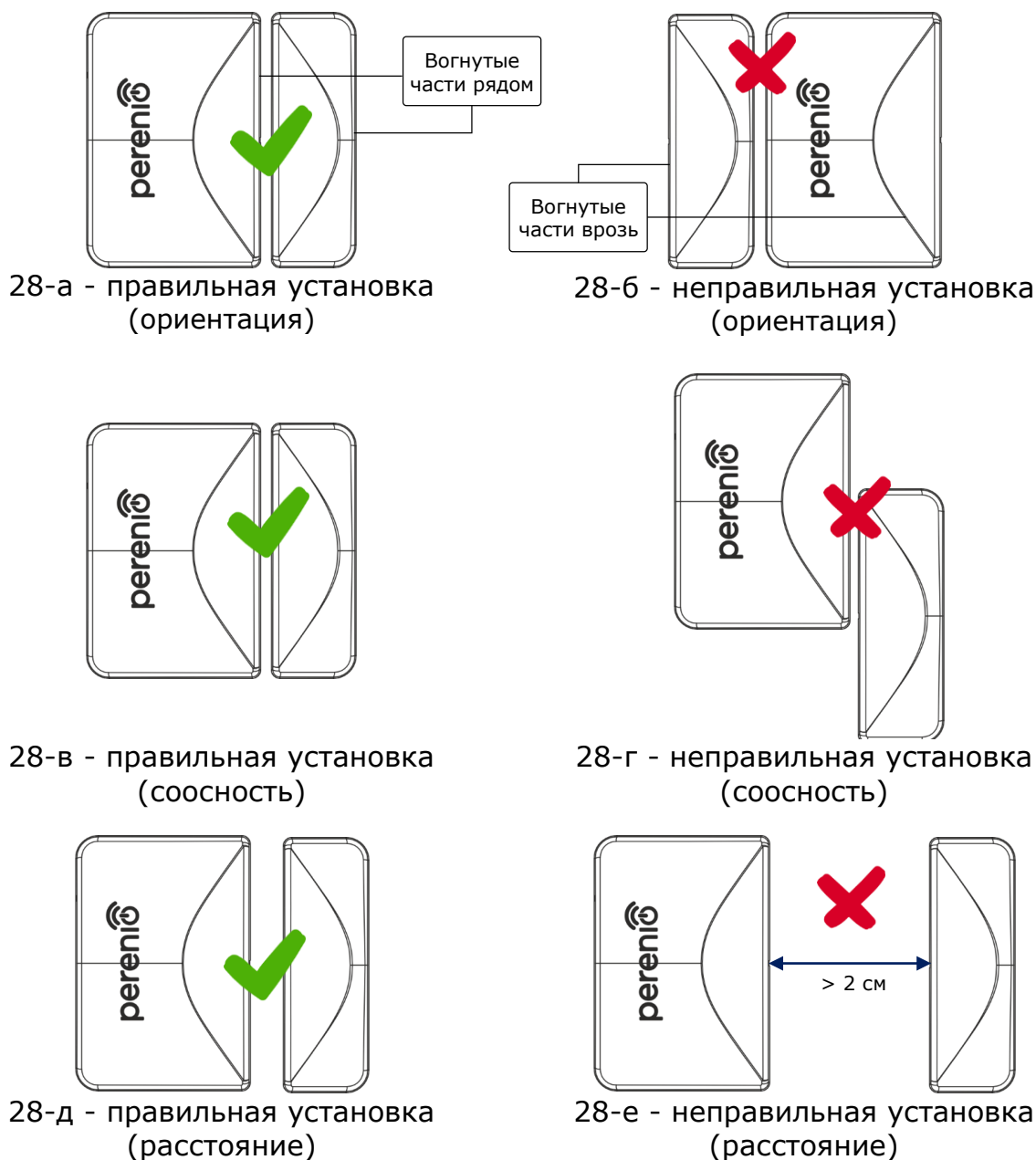
Рисунок 28 – Правила установки датчика и магнита
