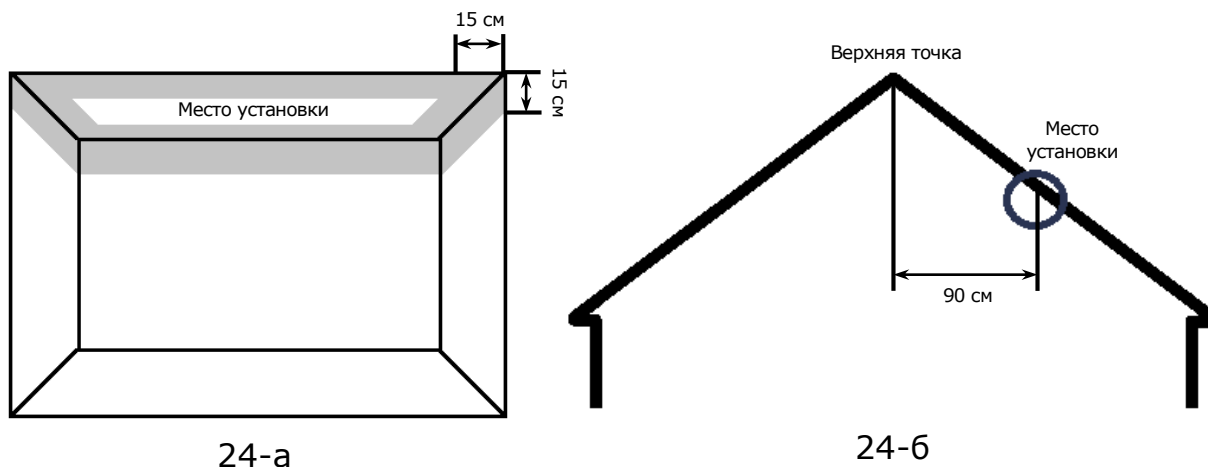
Рисунок 24 – Установка датчика дыма на плоский/скошенный потолок
