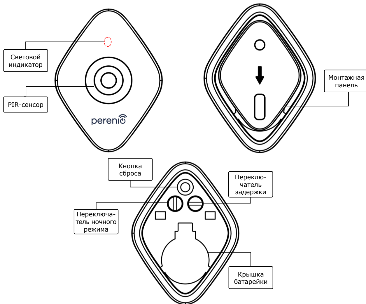
Рисунок 14 – Составные части датчика движения PECS01
