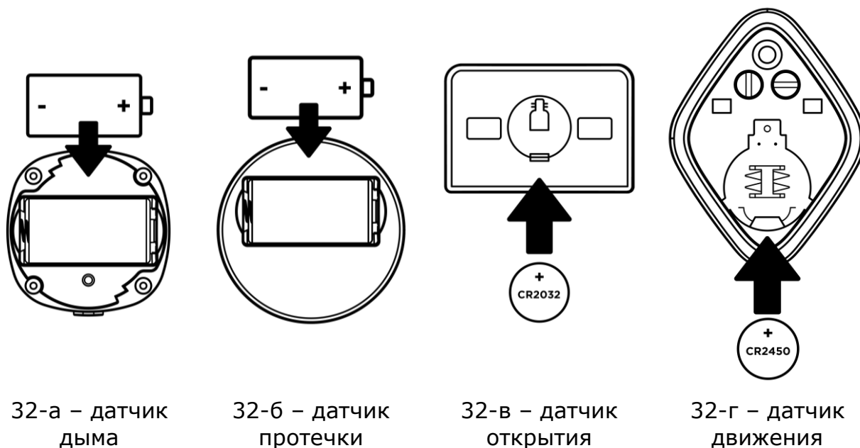
Рисунок 32 – Ориентация батарейки при вставке в датчики
