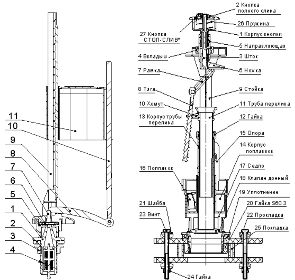
Рис. 1 Арматура наполнительная .
