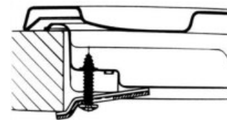
Крепление варки высотой 20 мм с помощью болта
