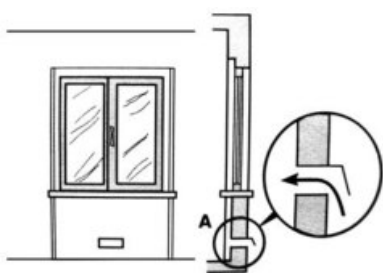
Рис. А Прямой приток воздуха через воздуховод
