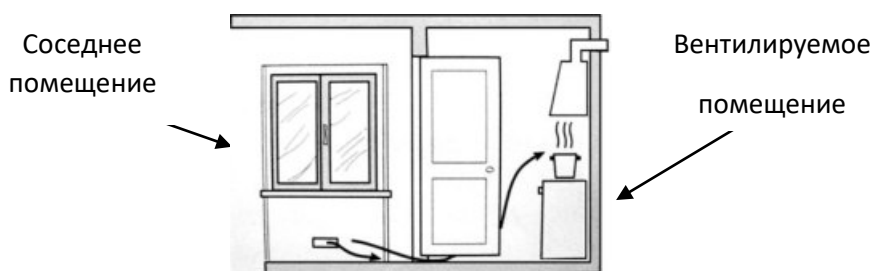
Рис. В Косвенный приток воздуха с увеличением вентиляционной щели между окном и полом
