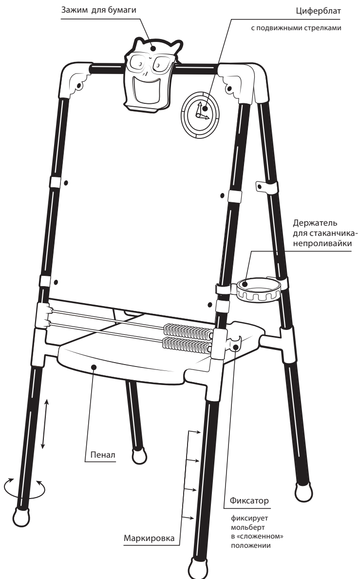
Рис. 1 Мольберт в разложенном виде
