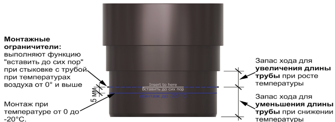
Рис. 32 Предохранительная система водоотведения на фитингах BC PREMIUM и STANDARD
