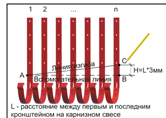
Рис. 13 Разметка кронштейнов для последующего изгиба
