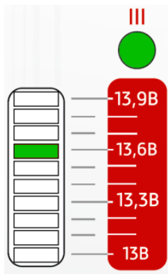
Рисунок 5 – Настройка напряжения третьей стадии, равного 13,6 В
