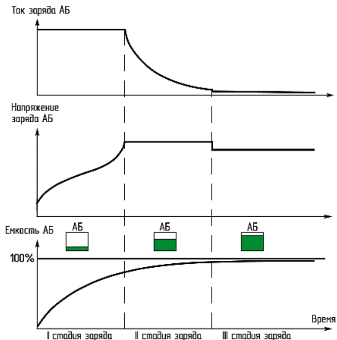
Рисунок 2 – Трехстадийный процесс заряда аккумуляторной батареи
