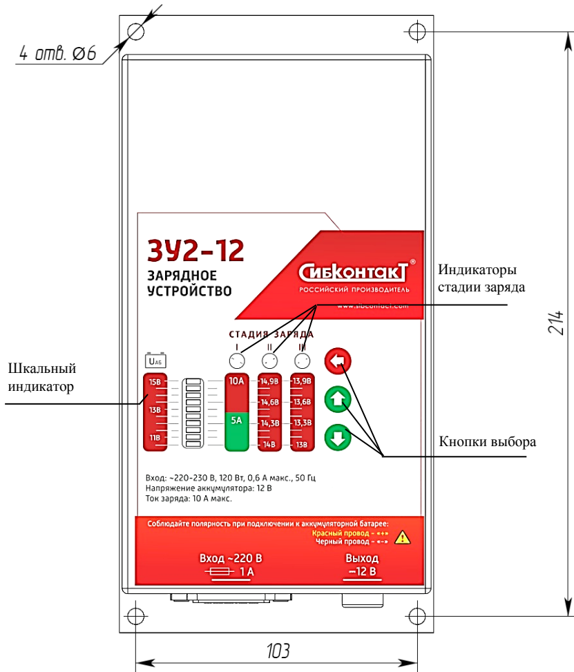
Рисунок 1 – Внешний вид лицевой панели и установочные размеры зарядного устройства
