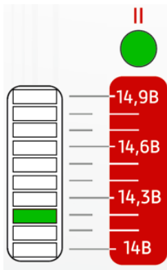
Рисунок 4 – Настройка напряжения второй стадии, равного 14,2 В
