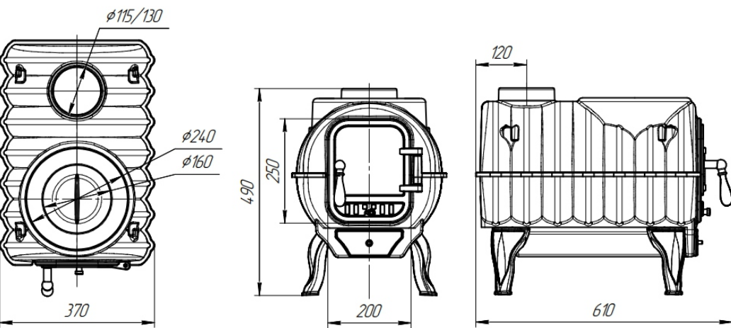
Общий вид печи «Тайга Про»
