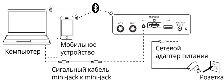
Рис.3. Схема подключения
