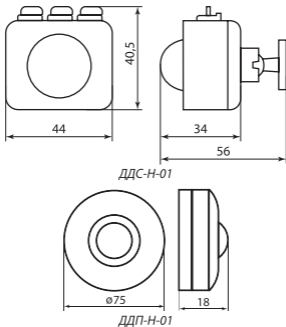
Рисунок 1. Габаритные и установочные размеры датчиков, мм
