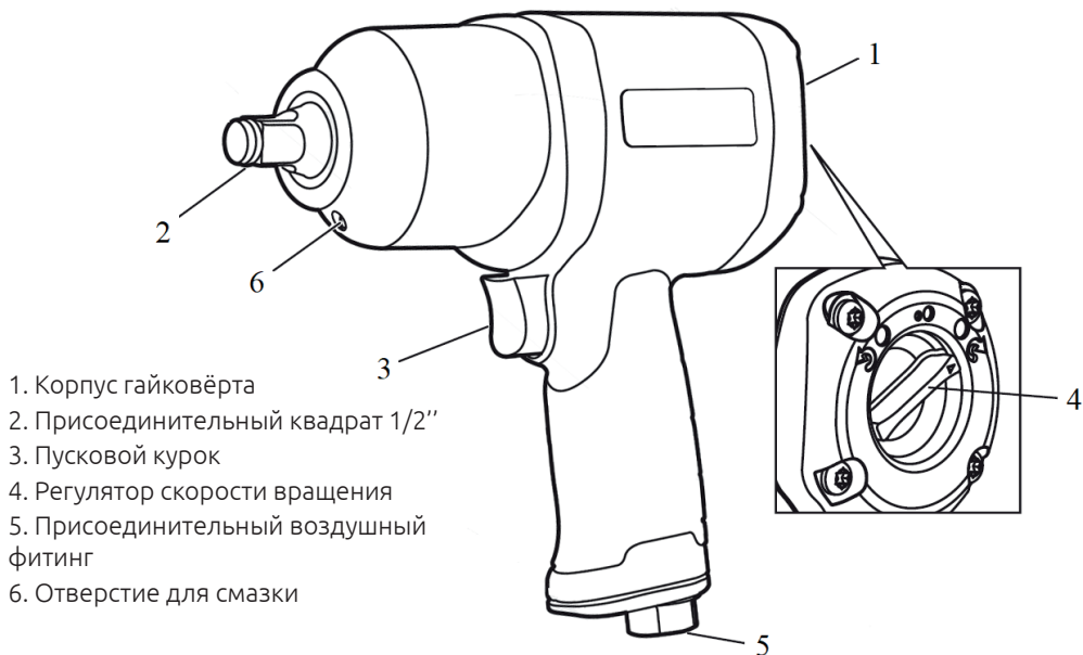
Рис. 1. Основные элементы пневматического гайковёрта «ПУЛЬСАР»
