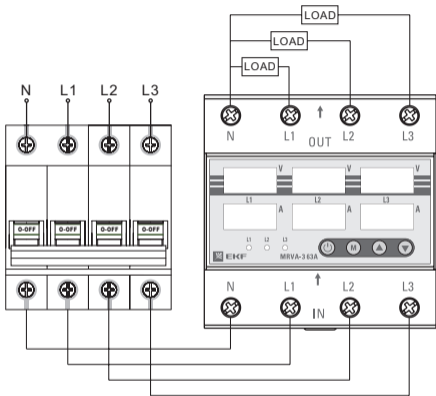
Рис. 14 Схема подключения
