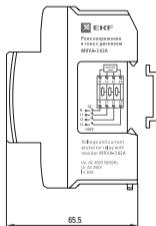
Рис. 15 Габаритные и установочные размеры
