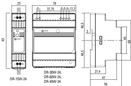
Рис. 2 Габаритные размеры блока питания.
