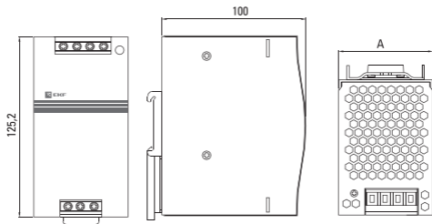
Рис. 3 Габаритные размеры блока питания DR-75W-24, DR-120W-24, DRP-240W-24.
