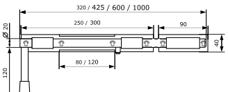
Засов универсальный ЗУ-400 мод.2
