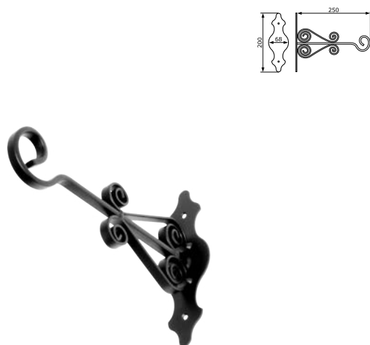
Кронштейн для кашпо мод. 10 25 см
