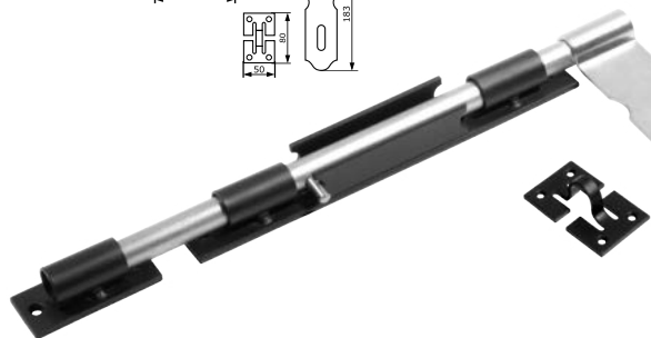
Засов ДОБРЫНЯ мод.2 (с накладкой) 300 мм / 450 мм / 600 мм
