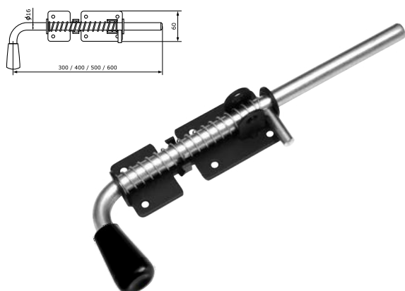
Засов с пружиной (с проушиной) 300 мм / 400 мм / 500 мм / 600 мм
