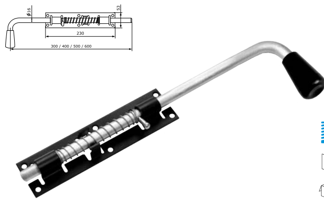
Засов с пружиной ЗСП мод.4 300 мм / 400 мм / 500 мм / 600 мм
