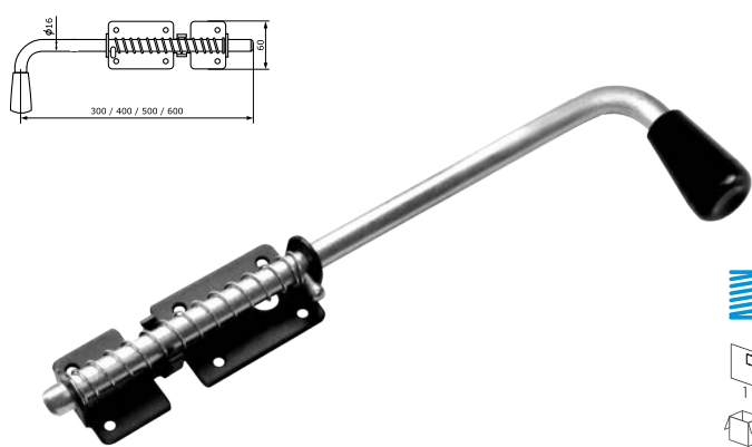
Засов с пружиной мод.3 300 мм / 400 мм / 500 мм / 600 мм
