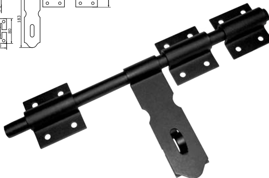
Засов ДОБРЫНЯ универсальный (с накладкой) 450 мм
