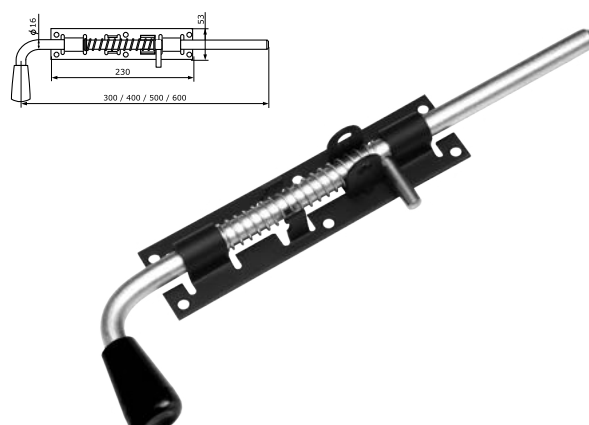
Засов с пружиной ЗСП мод.2 (с проушиной) 300 мм / 400 мм / 500 мм / 600 мм
