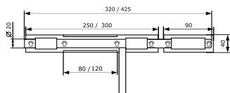
Засов воротный ЗВ-300 (с проушиной)
