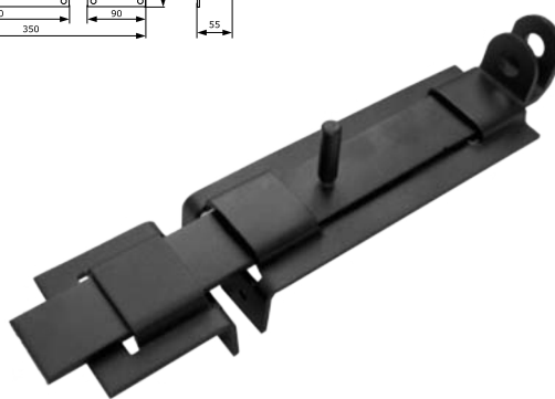
Засов с проушиной плоский ЗПП-350 мод.2
