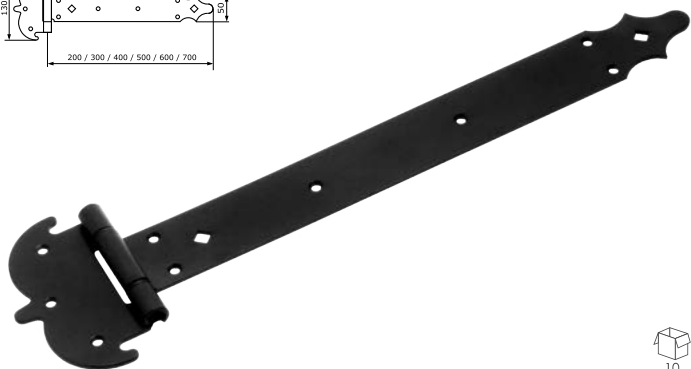
Петля-стрела фигурная мод.4 ПС-200 / 300 / 400 / 500 / 600 / 700
