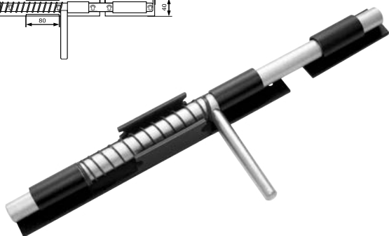
Засов ДОБРЫНЯ с пружиной 300 мм
