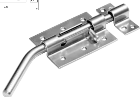
Засов гаражный ЗГ-100
