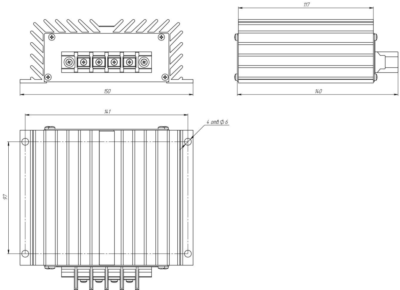
Рисунок 2. ПН1-50 общий вид
