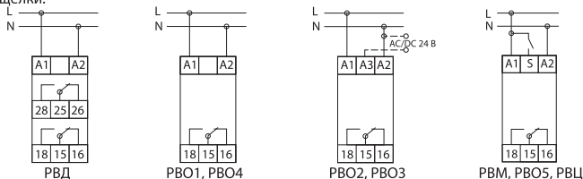
Рисунок 2. Схемы подключения реле к электрической сети
