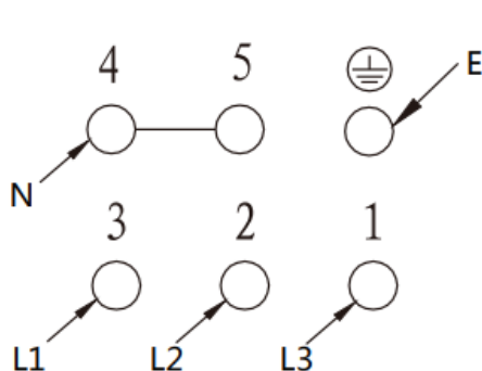
Трёхфазное, 380-415 В, ~50/60 Гц
