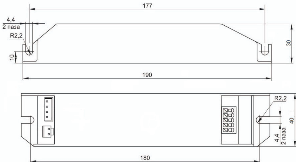
Рисунок 1 – Габаритные размеры БАП
