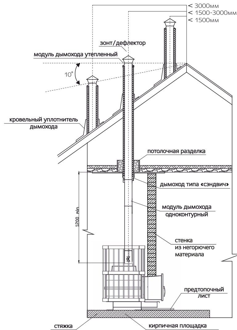
Рис. 3. Схема установки печи Kennet Бастион 22, вид сбоку
