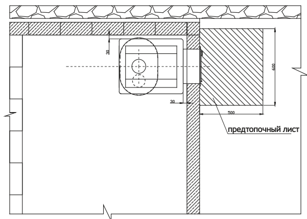
Рис. 4. Схема установки печи Kennet Бастион 22, вид сверху
