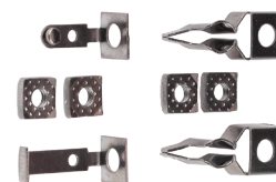
Контактные группы розетки и выключателя для алюминиевой проводки (хромирование)
