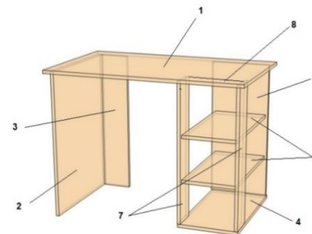
Схема сборки стола
